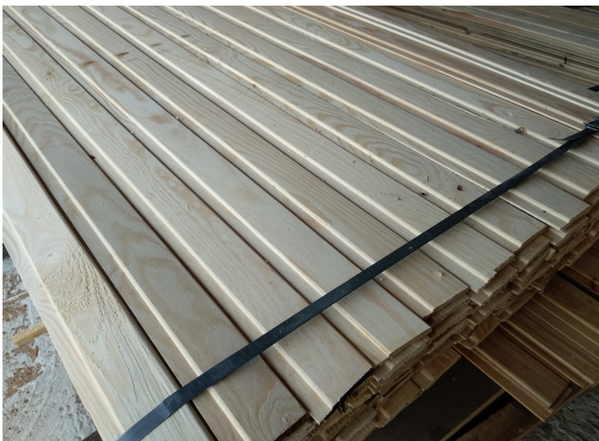
Детали профильные из древесины (доска для покрытия пола ДП-27, доска для покрытия пола ДП-35, плинтус ПЛ-6, наличник Н-1, обшивка О-2, обшивка (блокхаус)) СТБ 1074-2009
